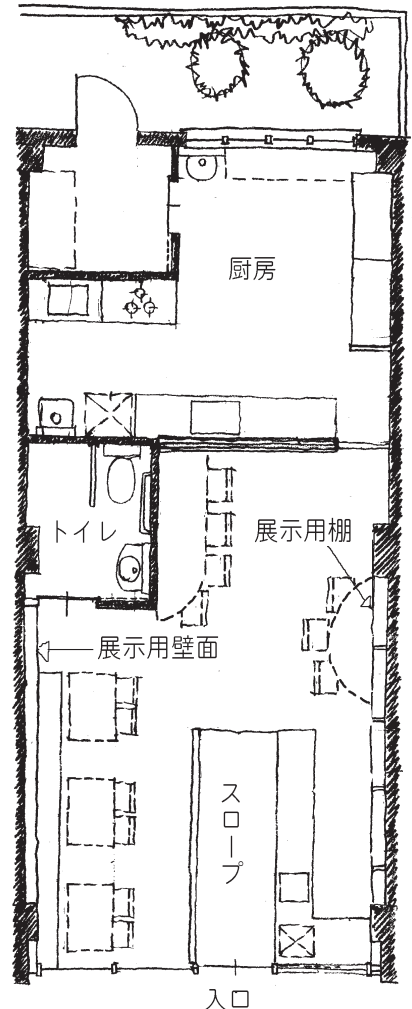
まんまん堂 平面図
